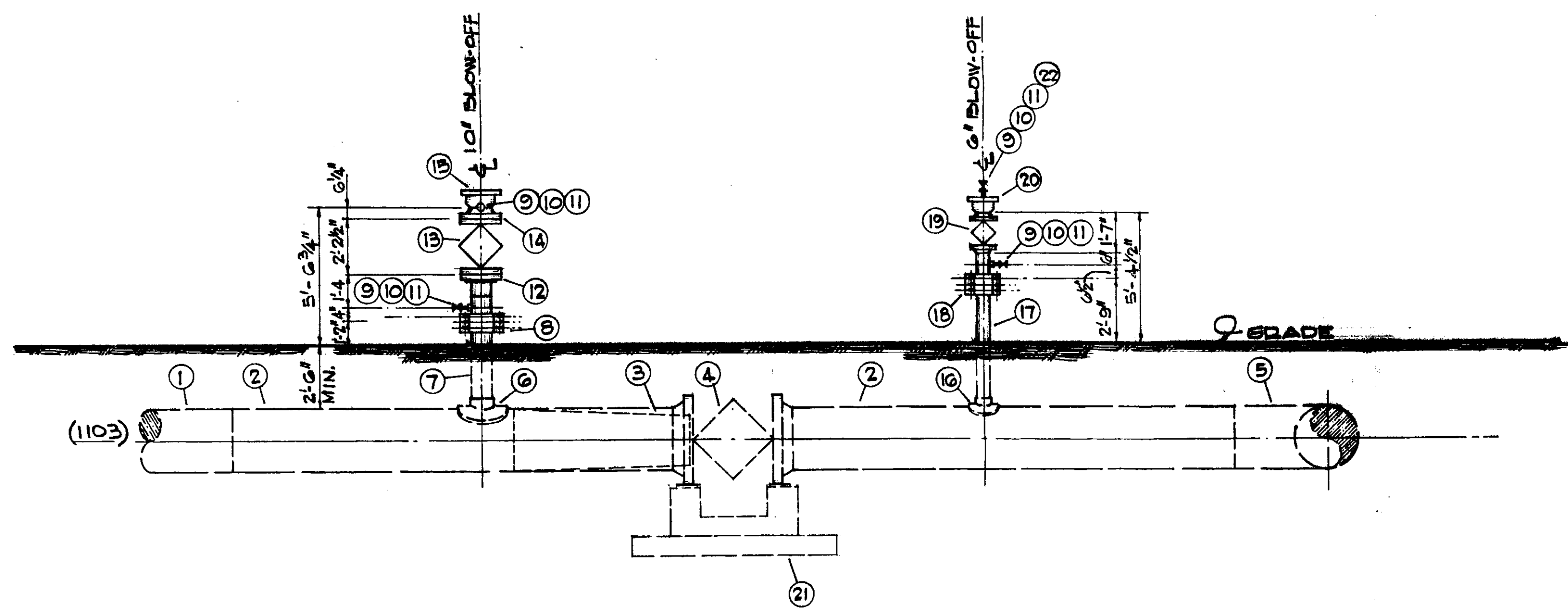
ELEVATION B-B
